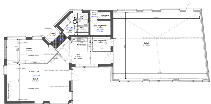
PLAN PROJET échelle 1/75°
